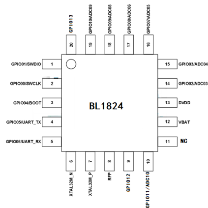
图 2.2 BL1824 QFN20 管脚定义
