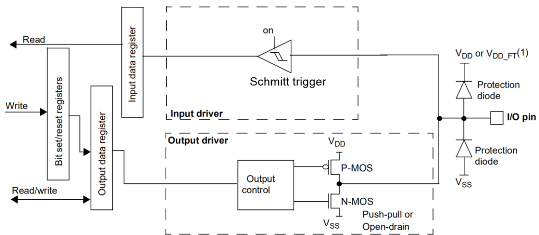
图 6.10 输出配置
