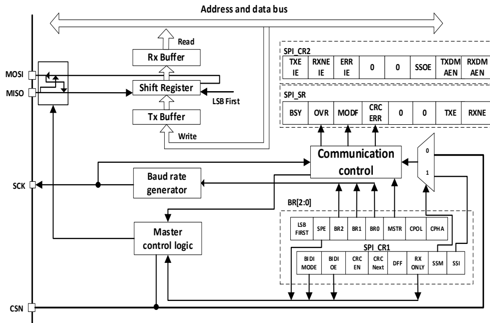
图 6.15 SPI 框图
