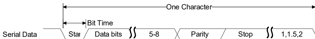
Figure 6.12 串行数据格式
