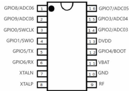
图 2.1 BL1824 SOP16 管脚定义
