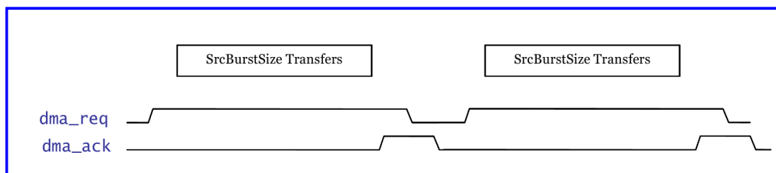
图 6.2 硬件握手实例
